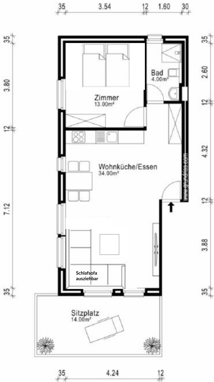
Erdgeschoss
